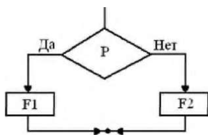
Рис. 2. Ветвление
