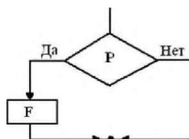
Рис. 3. Неполное ветвление
